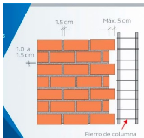
Figura 19: Espesor del mortero entre ladrillos
