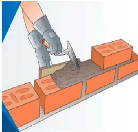
Figura 17: Distribución de mezcla
